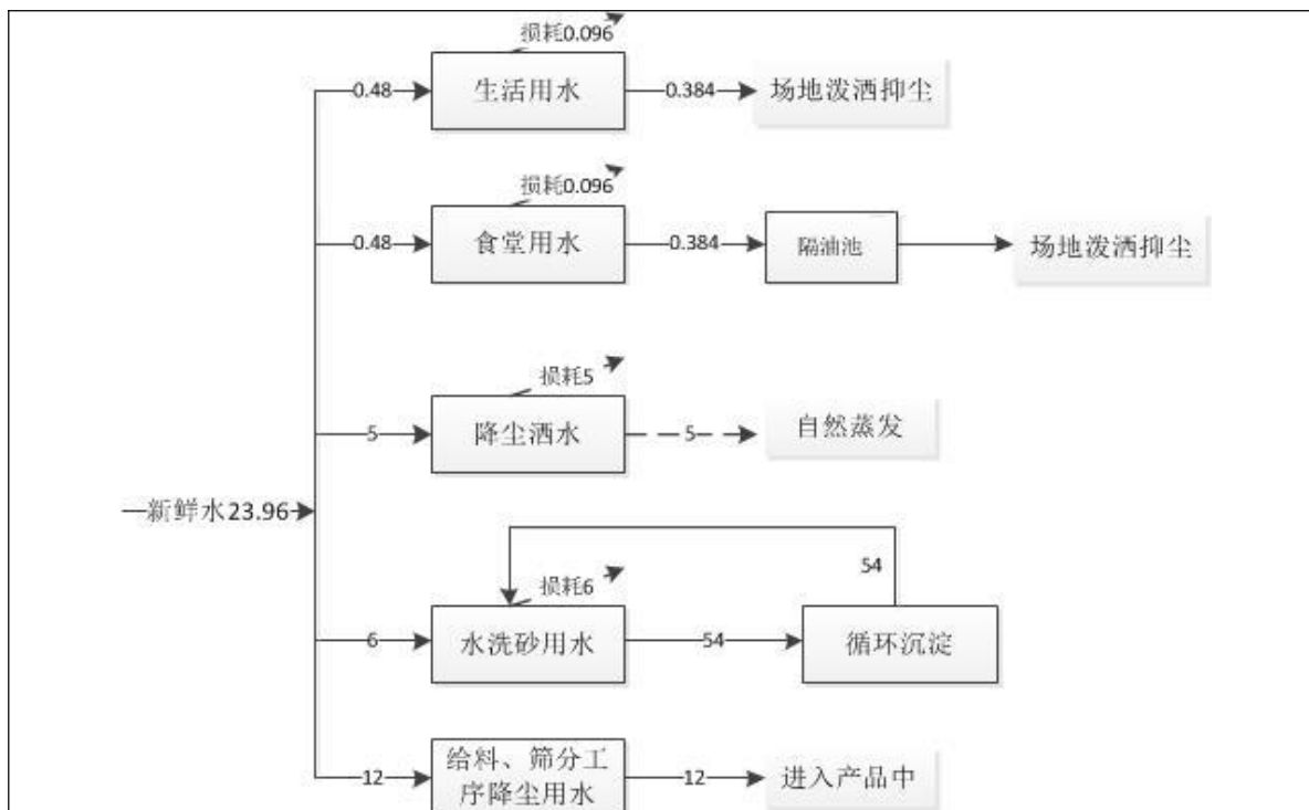
图 2--3 项目供排水平衡图
